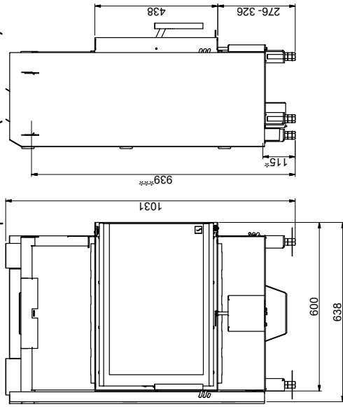
Dibujos con dimensiones Scan 5003, con escudo térmico para aislante (Accessorio)
