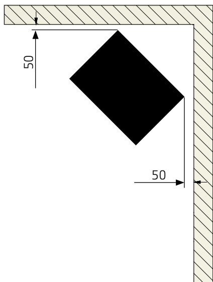
Colocación en rincón a 45°
