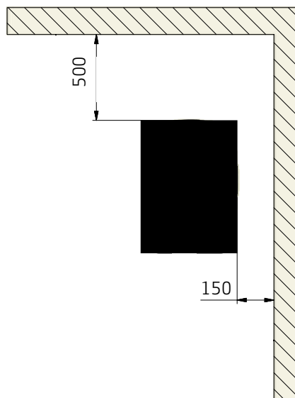
Instalación paralela a la pared posterior
