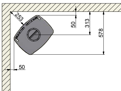
65-1, 65-3, 65-7 y 65-9 (sin ventanas laterales) Instalación de esquina de 45°
