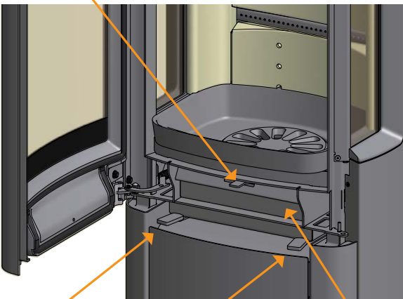
Aire primario Aire secundario Cajón de cenizas
