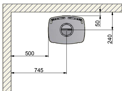
65-2, 65-4, 65-8 y 65-10 (con ventanas laterales) Instalación paralela
