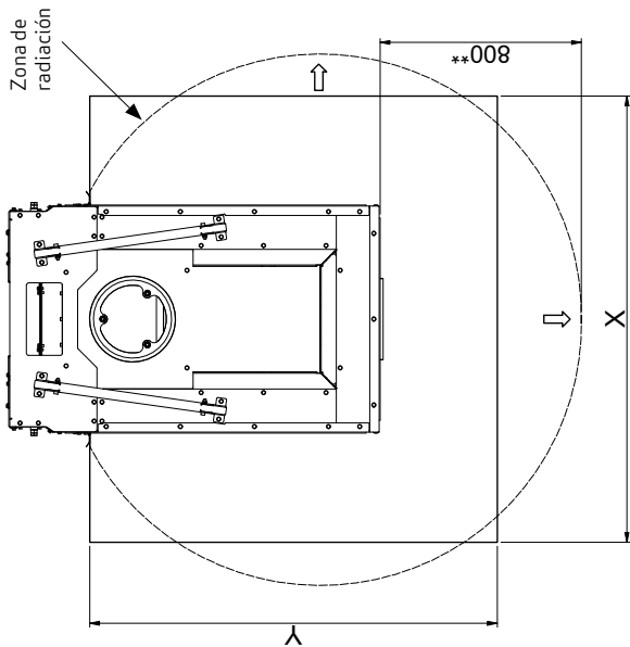
Placa de suelo
