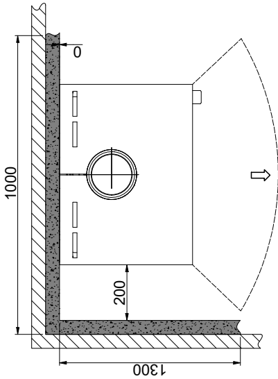
Distancia mínima a una pared de material combustible protegida con cortafuegos
